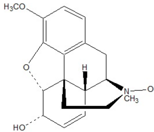
Codeine N-Oxide
