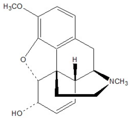
Codeine
